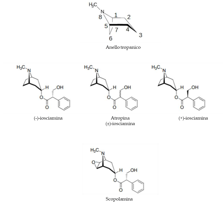
Figura 1. Formule di struttura, dall'alto: anello tropanico; (-)-iosciamina, atropina e (+)-iosciamina, (-)-scopolamina
